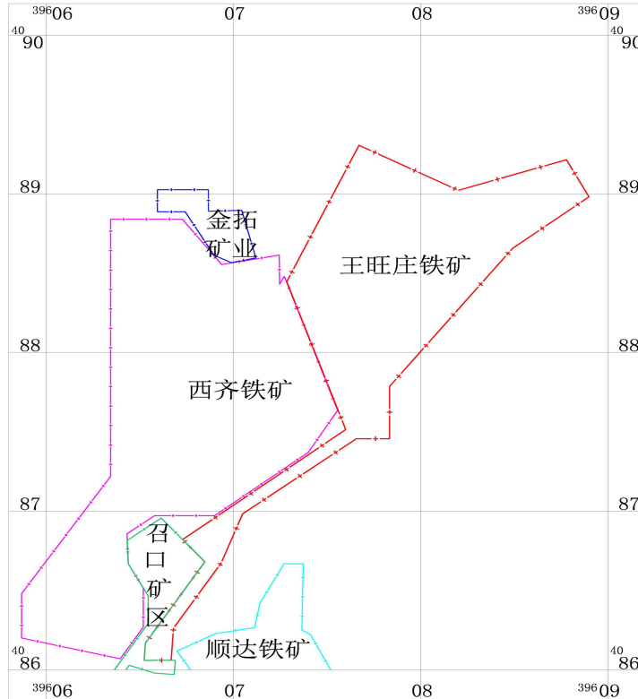
图 5-1 四邻关系图
